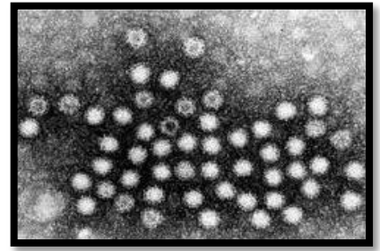
ノロウイルスの電子顕微鏡写真
